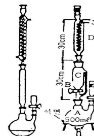
수은분해장치의 예
