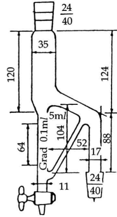
(a) 물보다 비중이 큰 기름용 증류두 : Clevenger Traps(단위 : mm) (b) 물보다 비중이 작은 기름용
