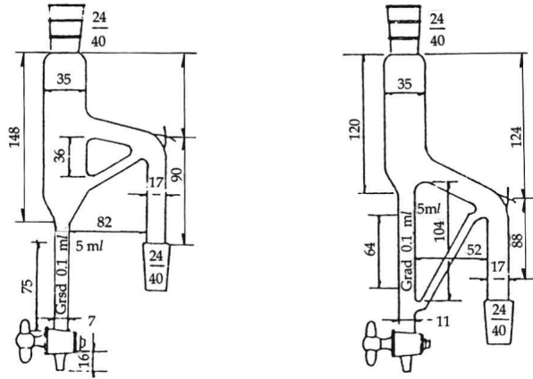
증류두 : Clevenger Traps(단위 : mm)
