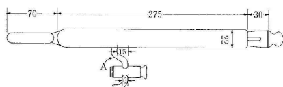
테리히관 (규격 : mm)
