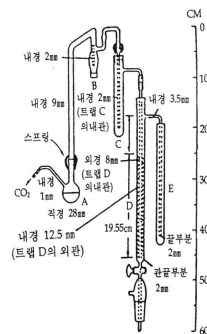
옥시에틸렌 정량장치
