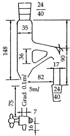
(a) 물보다 비중이 큰 기름용 증류두 : Clevenger Traps(단위 : mm) (b) 물보다 비중이 작은 기름용
