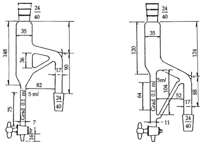
증류두 : Clevenger Traps(단위 : mm)
